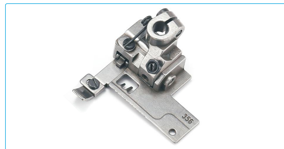
名称: 压脚(356) Description: Presser Foot (356) 代 码/Part NO: 30116005 适 配: W4S/ K5/W4/ K4系列 02BB/23BB机型 Machine Type: 02BB/23BB type for W4S/ K5/W4/ K4 series
