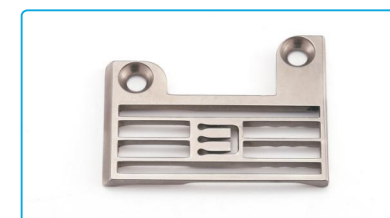
名称: 针板(01CB)(356) Description: Needle Plate (01CB, 356) 代码/Part NO: 30715004 适配: 8670系列-01CB机型 Machine Type: 01CB type for 8670 series
