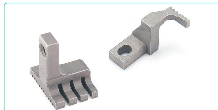
名称: 牙齿组件 Description: Feed Dog 代 码/Part NO: 30214008 / 30214009 适 配: W4/W4S/K4/K5系列-02BB机型 Machine Type: 02BB type for W4/W4S/K4/K5 series
